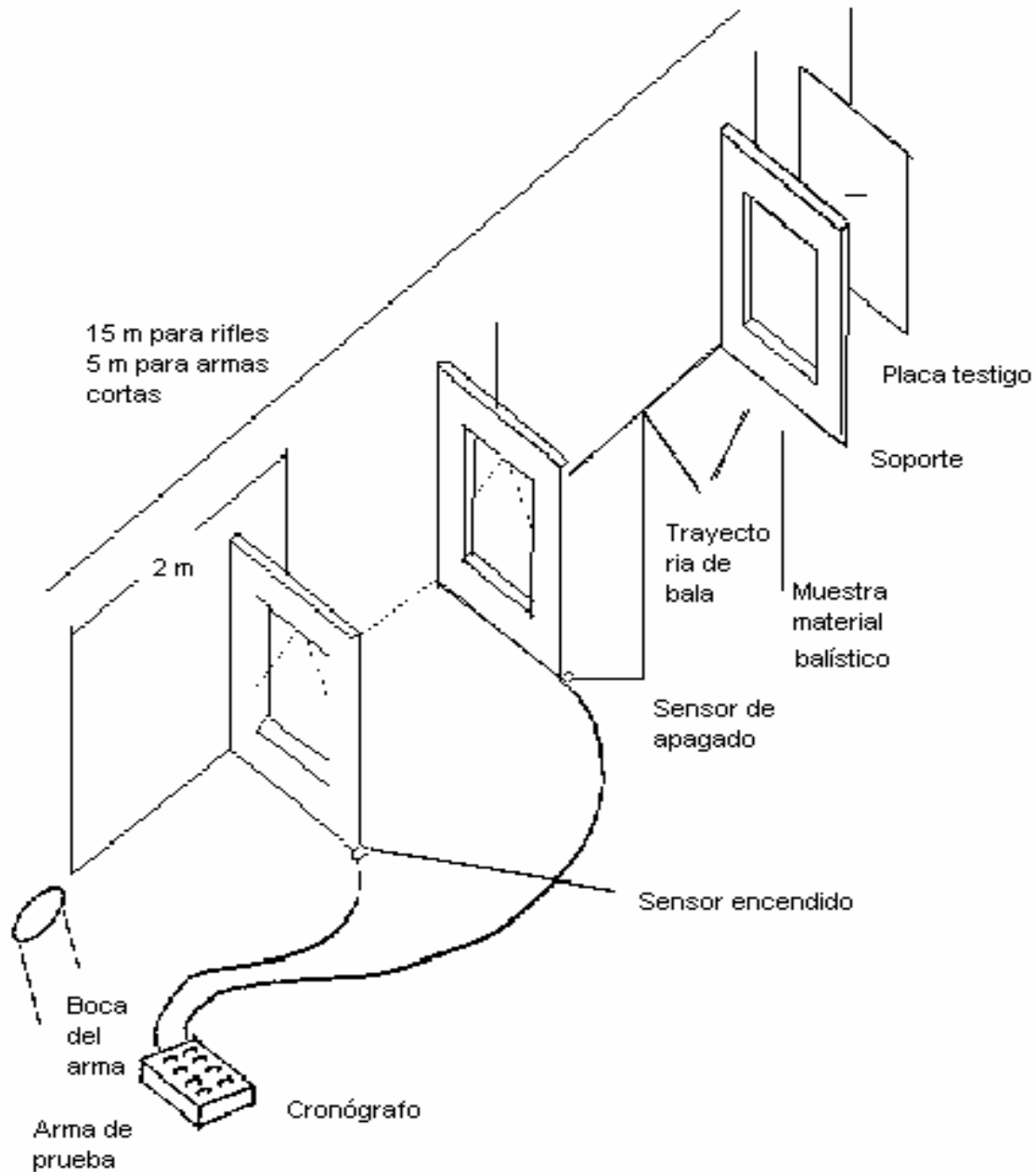
Figura 2.- Esquema ilustrativo para determinar el nivel de resistencia a los impactos de bala.
